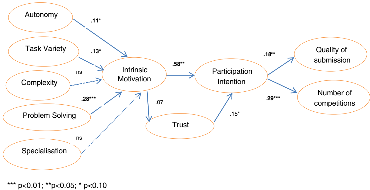
Fig. 2. Structural model. *** p < 0.01 ; ** p < 0.05 ; * p < 0.10 .
